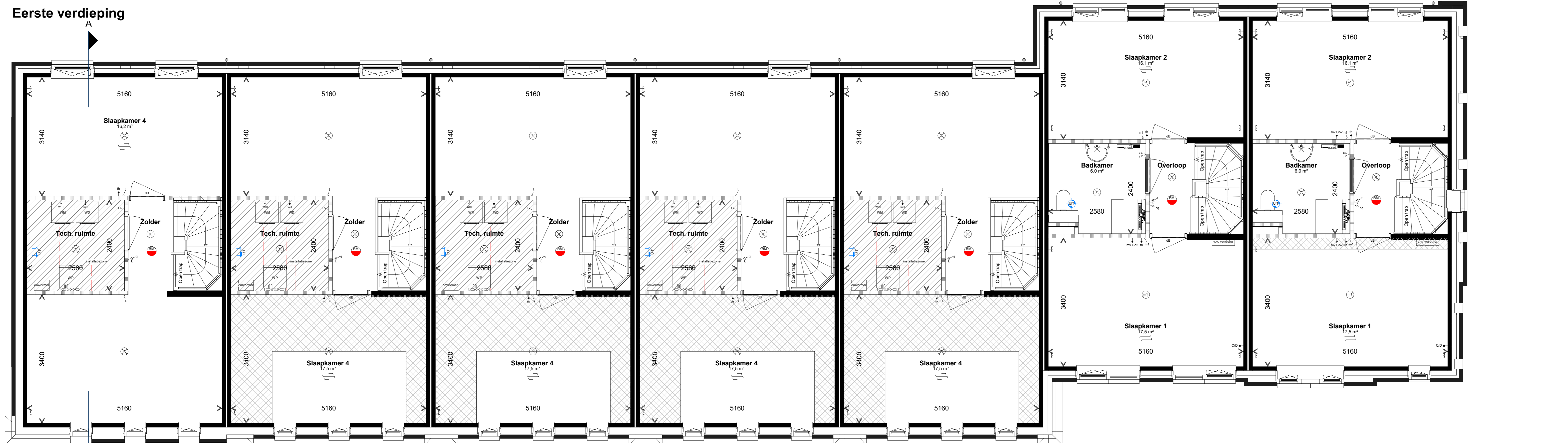
Eerste verdieping
